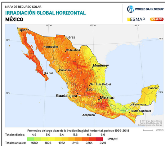
Figura 6: Mapa de la Irradiación Global Horizontal de México Tomada de: SOLARGIS (2019a).
