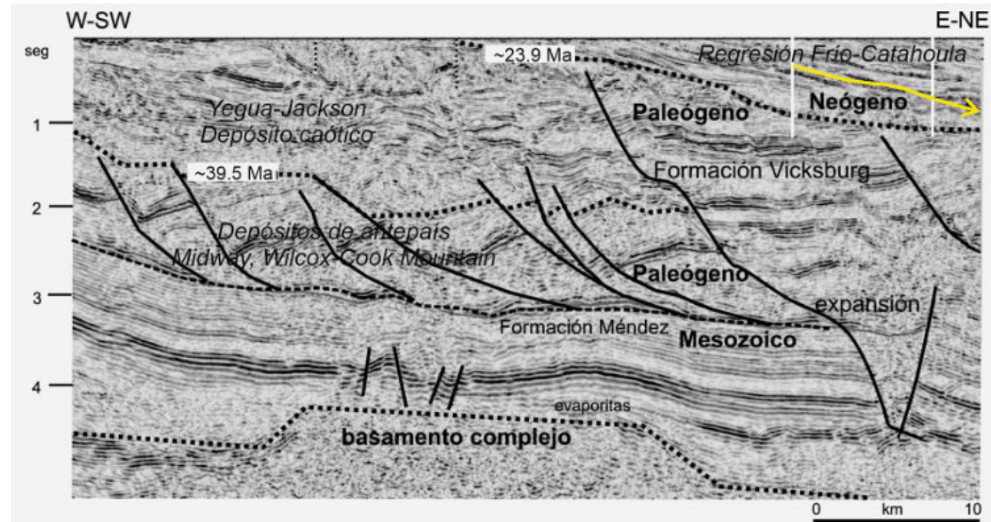
Figura 2. La sección sísmica regional muestra las discordancias relevantes como límites de secuencia (~39.5 y ~23.9 Ma). Explicación en el texto.
