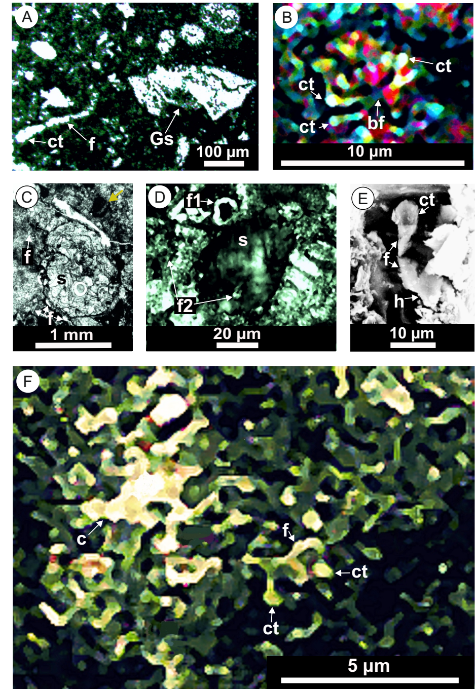
Fig. 4. Filamentos microbicos de la Formación Cacarajícara (Sierra del Rosario): A – El filamento uniserial grande (235 µm de longitud y 15 µm de ancho), (ct) célula terminal (apical) cerca de 30 µm de ancho, (Gs) Globotruncanita stuarti (de Lapparent) redepositada de las capas del Campaniano-Maastrichtiano (muestra/sección delgada LP-CA-2, el corte de Lomas de Polier); B – (bf) Principal (o basal) filamento de una estructura microbica y filamentos microbicos (en forma de araña de luces) cerca de 5,2 µm de longitud, (ct) células terminales de algunos filamentos secundarios (muestra/sección delgada AP-47, Los Hoyos); C – (f) Filamentos uniseriales, 12-24 µm de ancho, situados cerca de una esférula espumosa de calcita (s) 1,7 mm de longitud y 1 mm de ancho. La flecha amarilla indica una esférula negra más pequeña (332 µm de longitud), muestra/sección delgada 6P-273; D – estructura microbica y filamentos microbicos que ocurren próximos a una esférula negra (s) 42 µm de ancho: (f1) filamento uniserial semicircular cerca de 16 µm de longitud y hasta 3,5 µm de ancho, (f2) numerosos filamentos ramificados 0,8-1,5 µm de ancho (muestra/sección delgada AP-64, el corte de Lomas de Polier); E – (f) Filamento uniserial (24x4 µm), ligeramente dañado en su parte media, (ct) célula terminal (apical), (h) célula basal (para adherir el filamento a otro objeto – “holdfast”), muestra/sección delgada PG-CA-1, el corte La Piedra de Genaro, la imagen del microscopio electrónico – un fragmento aumentado, de color falso); F – Densa red de los filamentos ramificados (muestra /sección delgada CP-67e, el corte tipo, la luz polarizada): (f) filamento principal, (ct) células terminales (apicales), (c) cemento calcáreo concentrado a lo largo de los filamentos.
