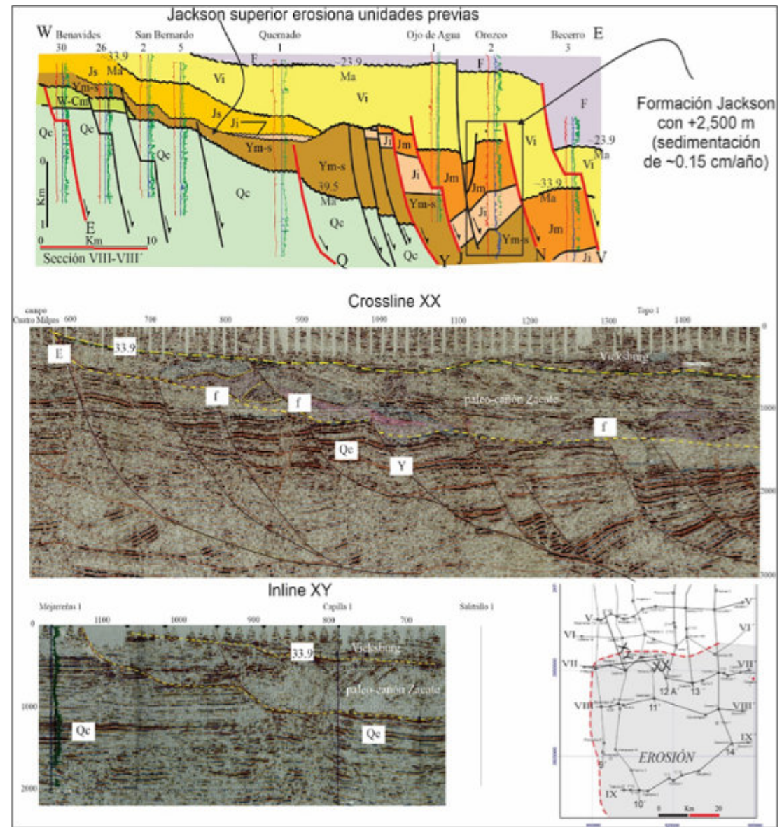
Figura 3. Datos de superficie y subsuelo indican una erosión profunda identificada como paleocañón submarino en el Eoceno tardío al sur de la Cuenca de Burgos. La Formación Yegua inferior y Jackson superior sobreyacen en discordancia a sucesiones previas en un área amplia.
