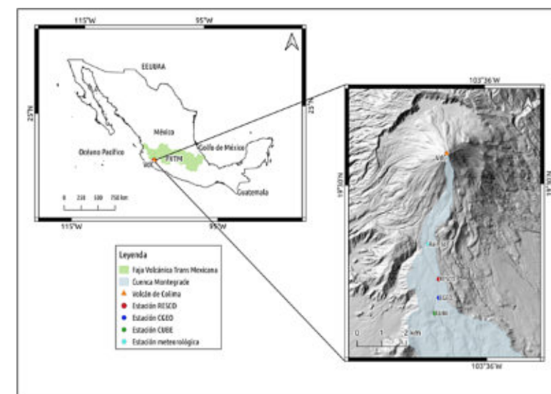
Figura 1.1. Localización del Volcán de Colima y estaciones de monitoreo.
