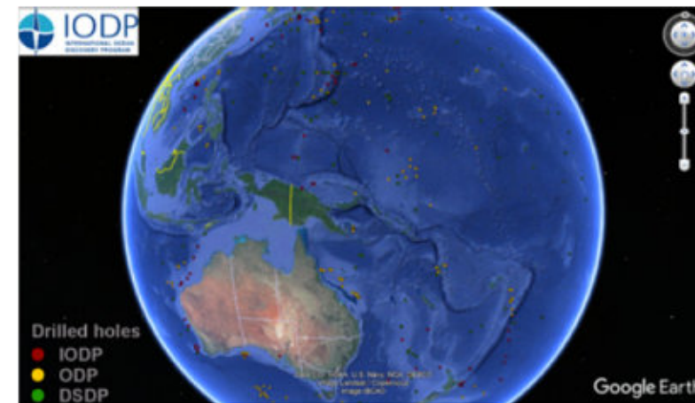
Visualización de todos los pozos en un archivo KMZ de IODP, ODP y DSDP (Extraído de: https://www.iodp.org/ )
