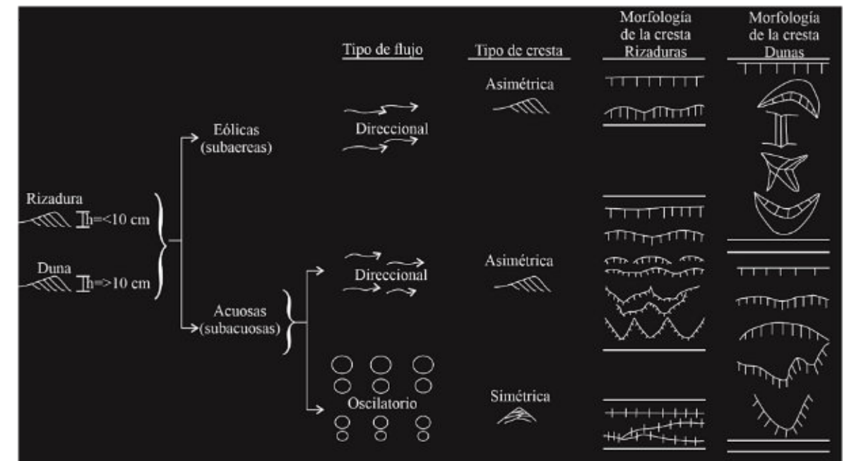
Fig. 2: Síntesis de los procesos de formación de las rizaduras y dunas, y sus formas resultantes. h= altura de la cresta.
