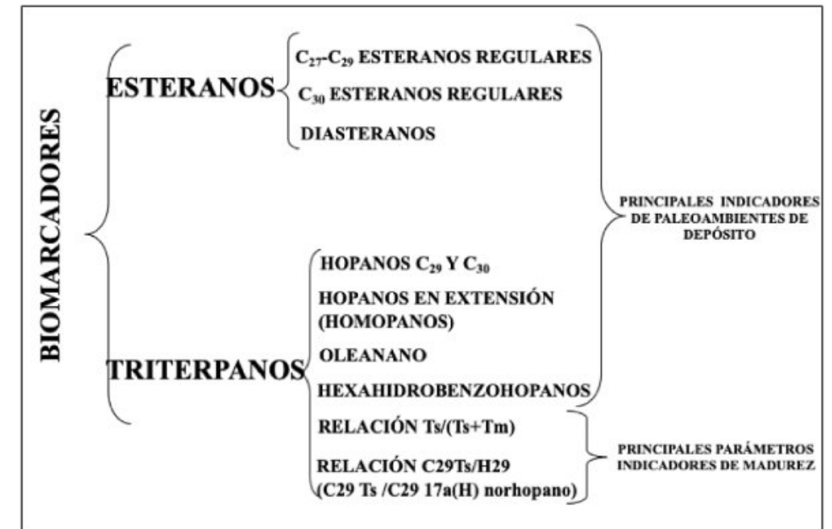
Figura 1. Muestra los principales Biomarcadores utilizados para determinar la madurez y el origen de los hidrocarburos.
