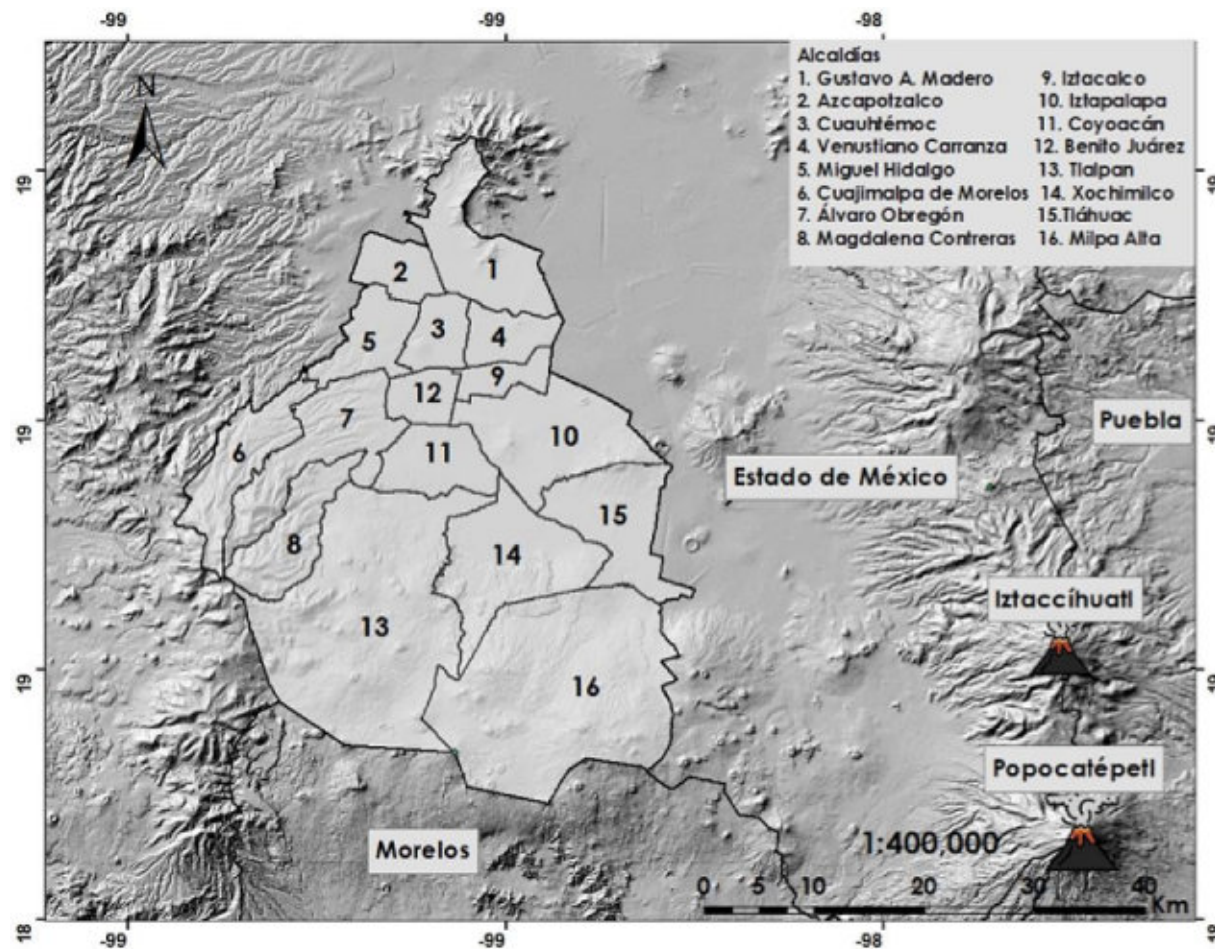
Figura 1.1. Área de estudio.
