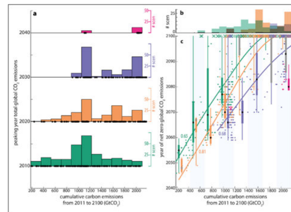
Figura 1: Influencia del año pico de emisiones globales de CO 2 en el momento de las cero emisiones netas de CO 2 globales. (a) Distribución de las emisiones de carbono acumuladas de 2011 a 2100 y año pico para las emisiones globales totales de CO 2 . (b) Distribución de escenarios que no lograron emisiones netas de CO 2 globales cero antes del siglo XXI. (c) Relación entre las emisiones de carbono acumuladas de 2011 a 2100 y el momento en que las emisiones globales de CO 2 alcanzan niveles de cero emisiones netas. Los colores verde, naranja, morado y rosa en los paneles (b) y (c) se refieren a los años pico que se muestran en el panel (a). Los puntos indican escenarios únicos. Los rombos muestran medianas, y los diagramas de caja y los bigotes indican el rango central de 50 y 90%, respectivamente, sobre cada contenedor sombreado. Los rombos vacíos indican que hay menos de 10 escenarios disponibles en un contenedor determinado y para un año pico determinado; los diamantes rellenos indican lo contrario. Los recuadros de colores indican que más del 80% de los escenarios realmente logran cero emisiones netas de CO 2 antes de 2100; cajas grises lo contrario. Las líneas diagonales en el panel (c) son líneas de suavizado sobre todos los puntos de datos para cada año pico, respectivamente. Los números en el panel (c) son valores R 2 para los ajustes respectivos Tomada de: Rogelj, J et al. (octubre 21, 2015).
