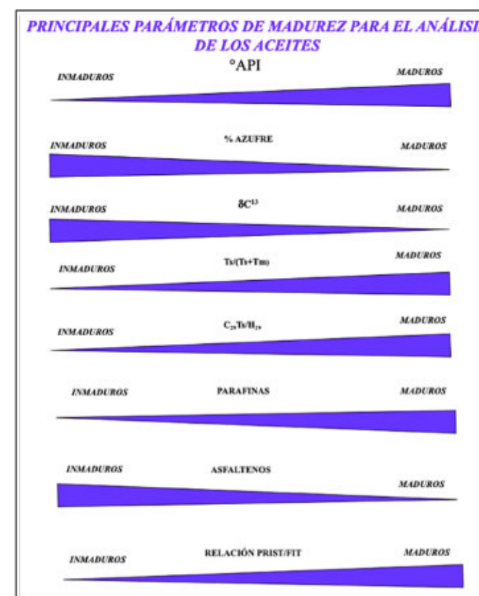
Figura 2. Muestra incrementos y decrementos de parámetros geoquímicos en función de su madurez.
