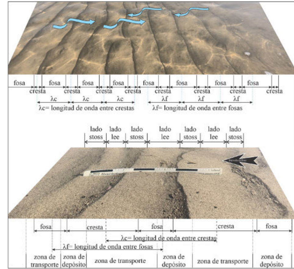
Fig. 1: Partes de las rizaduras generadas por flujos oscilatorios (imagen superior) y rizaduras desarrolladas por flujos direccionales (imagen inferior).
