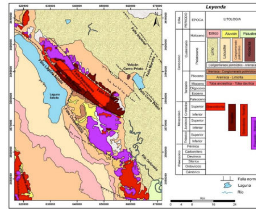
Figura 1.1. Mapa geológico regional para el campo geotérmico de Cerro Prieto (CGCP) (tomado de Macías-Vázquez y Rocha-López, 2013).
