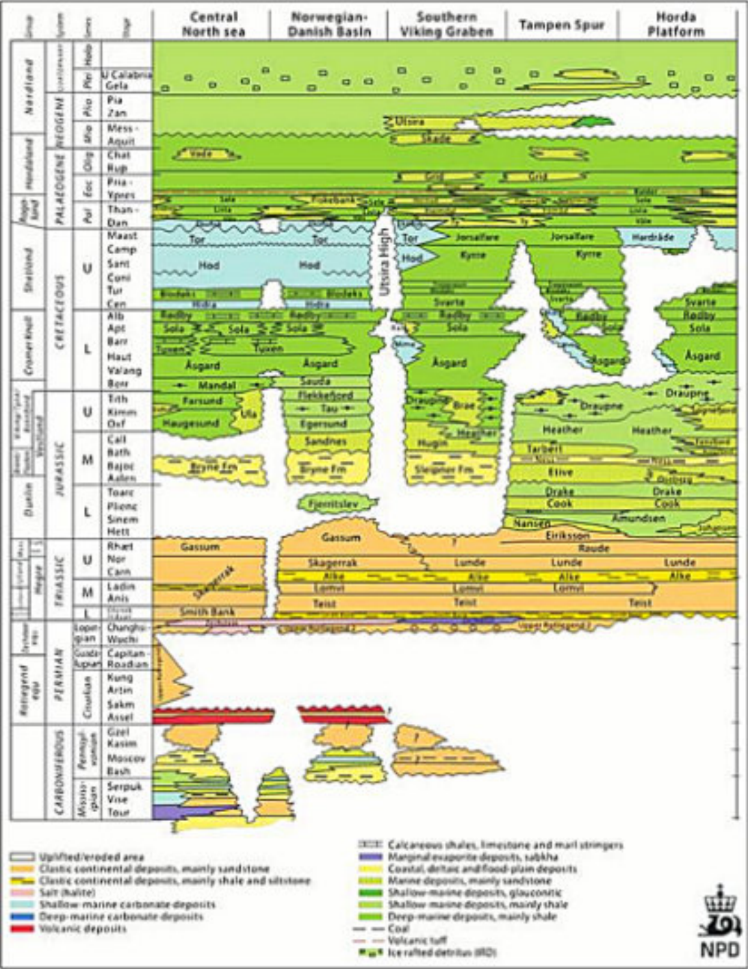
Figura #1. Columna Geológica del Estudio.
