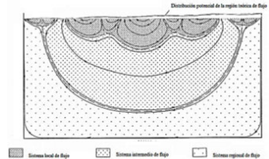
Fig. 8. Sistemas de flujo establecidos por Tóth (1963, ligeramente modificado).
