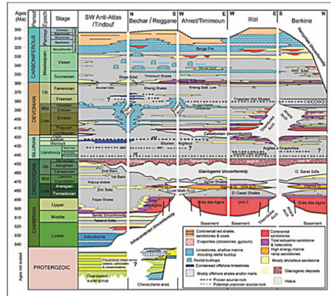
Figura 3. Tabla cronoestratigráfica de las cuencas del Sahara Argelino (Fuente: web de Alnaft).
