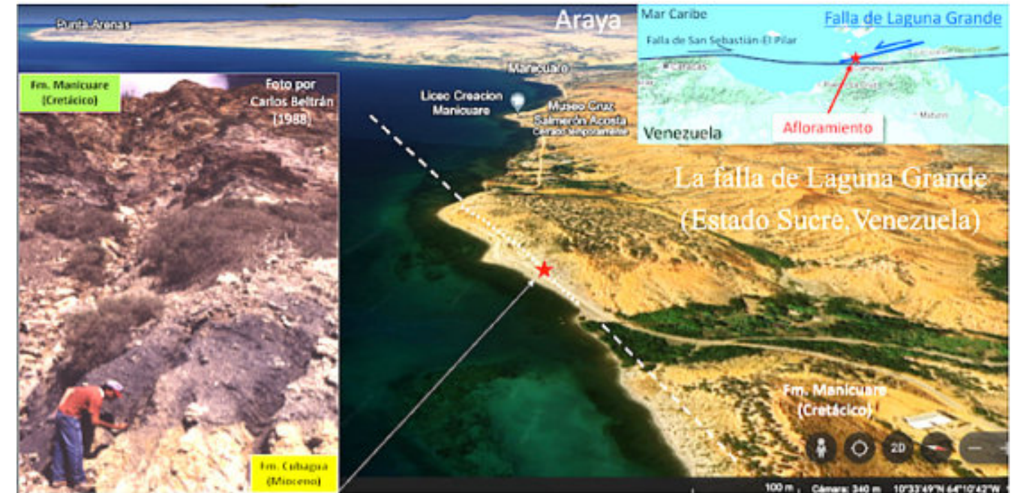
The Laguna Grande fault outcrop picture from 1988, and Google Maps satellite image ( Giraldo, 2024 ; Afloramiento de la falla de Laguna Grande (1988) e imagen satelital de Google Maps).
