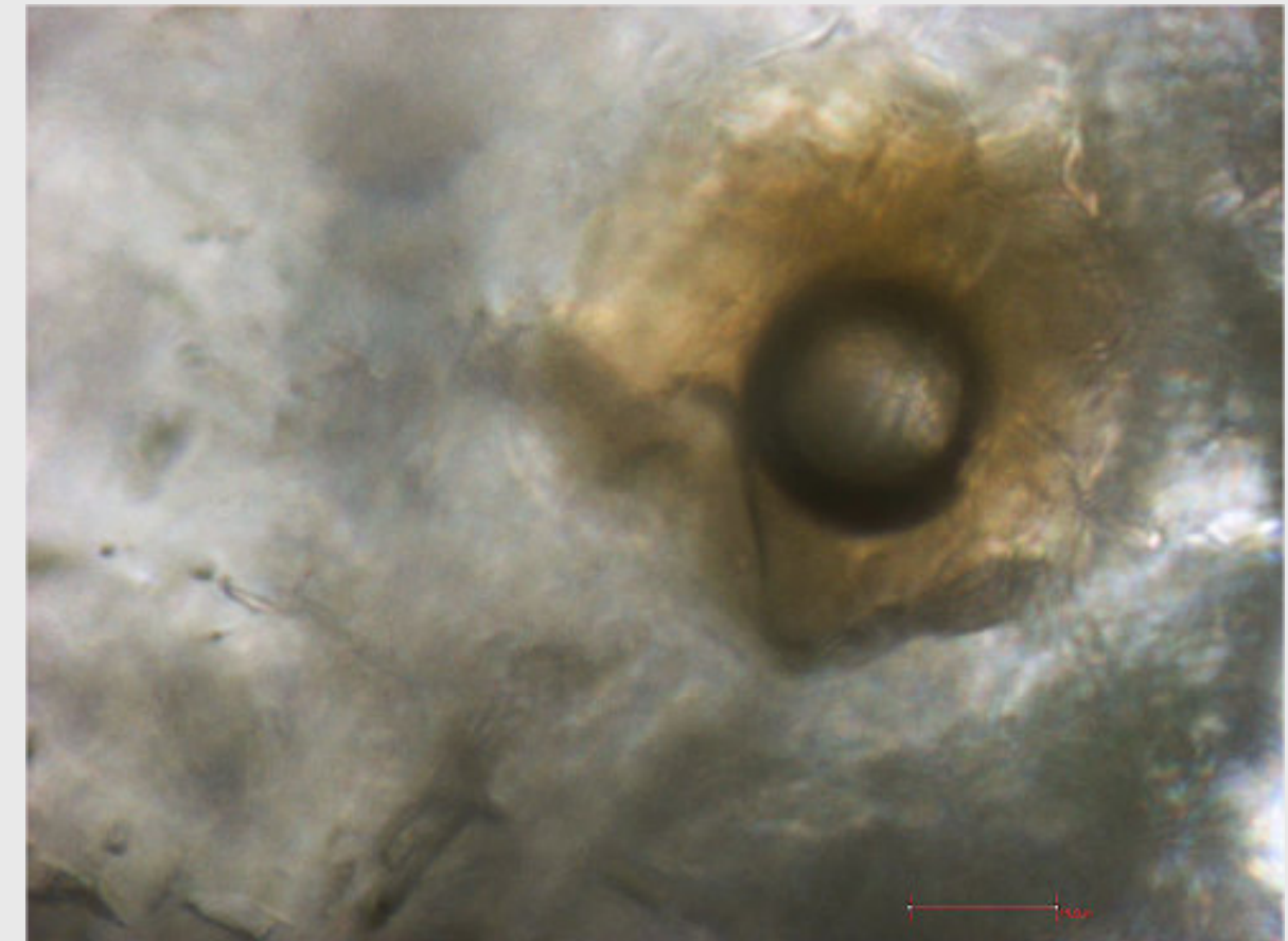
Inclusión fluida de hidrocarburo en luz paralela, Pérmico de Barents, Noruega.
